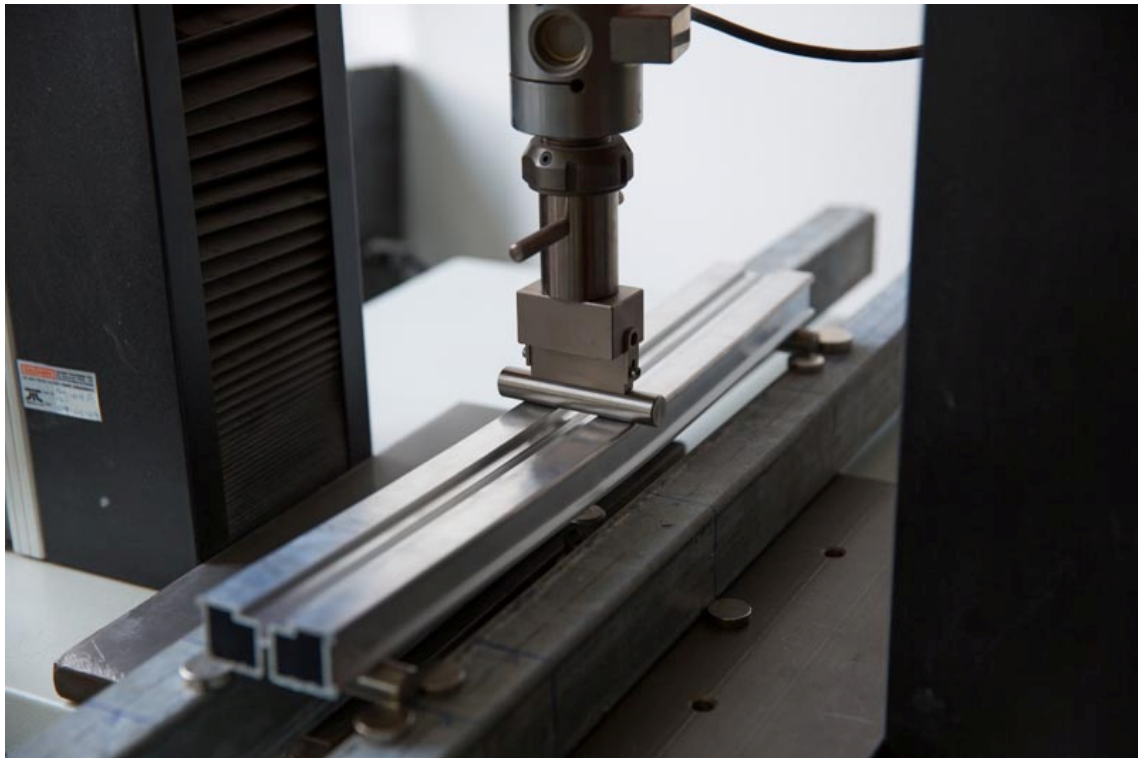
Fig. 1: test di flessione a tre punti / three-point bending test
